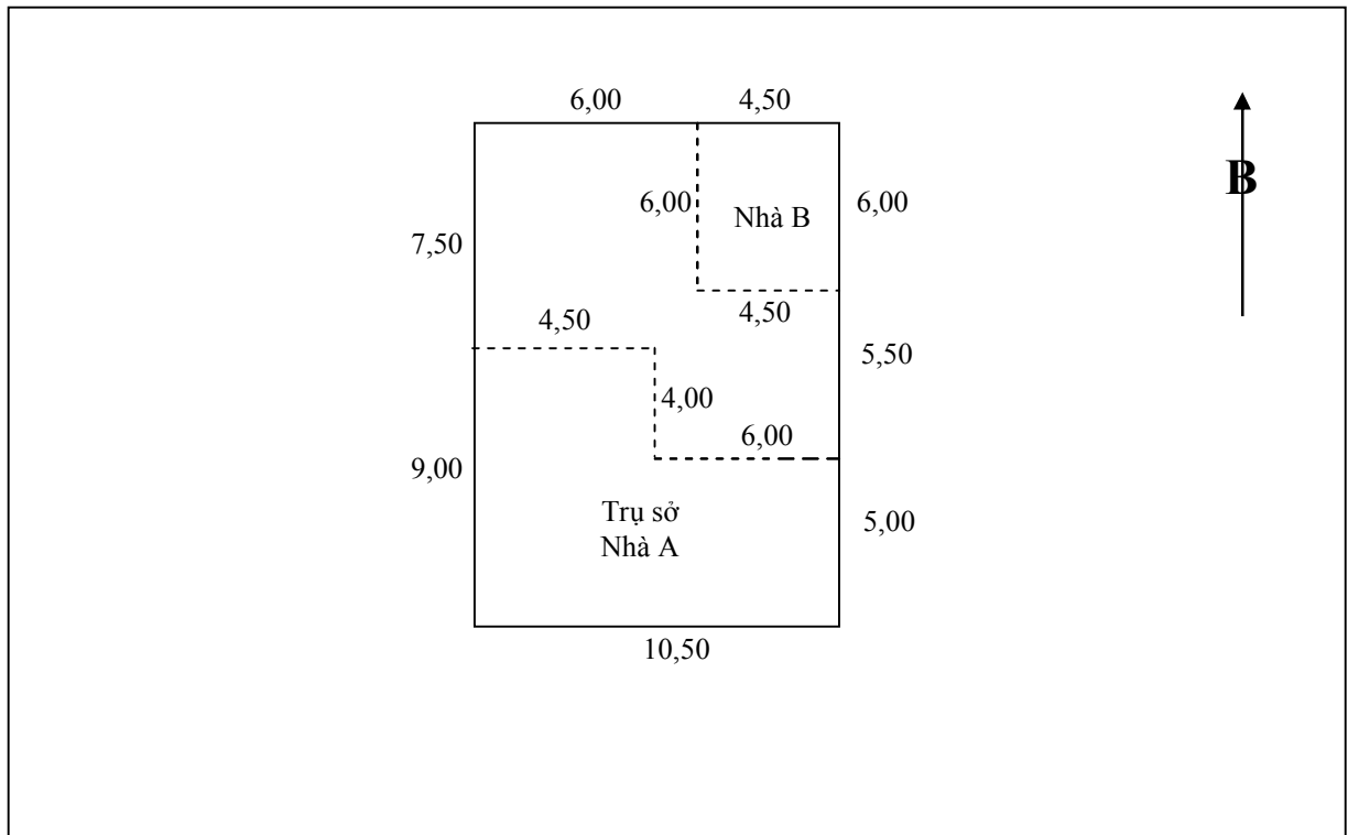
Hình 6. Sơ đồ thửa đất có công trình xây dựng
